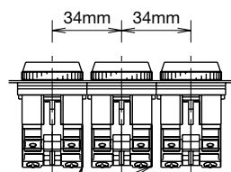
安全隔板 (HW-VU1型)
