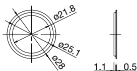
安裝孔尺寸圖
