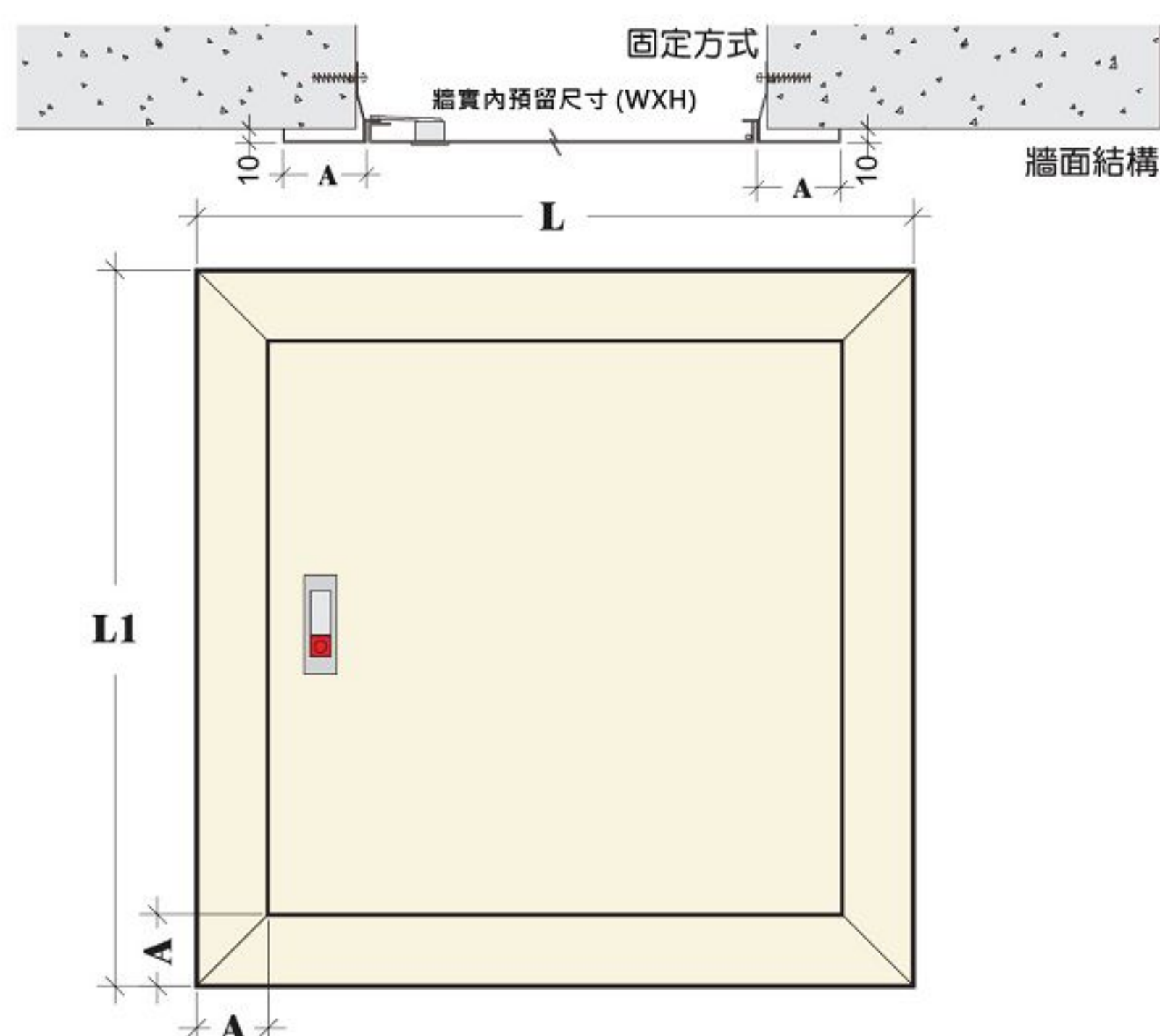
固定方式示意圖
