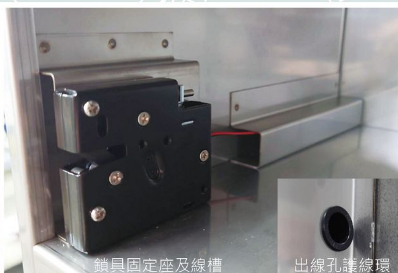
勾片固定座
