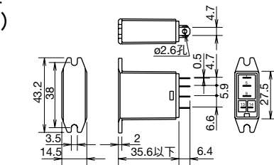
□DPDT 扁平端子型 (頂部凸緣安裝型)
