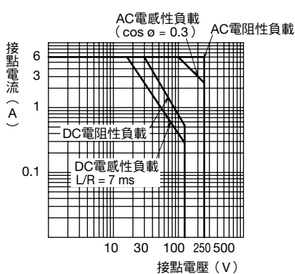
RU4 型（最大接點額定）
