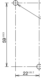
• 安裝孔加工圖
