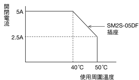
降低額定值遞減特性圖
