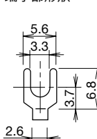
端子部形狀
