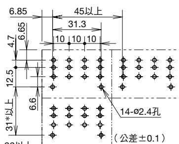
端子配置圖
