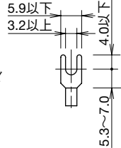
• 適用壓接端子
