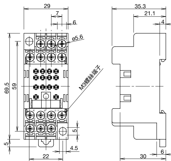
• 端子配置圖
