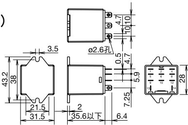
□4PDT 扁平端子型 (頂部凸緣安裝型)
