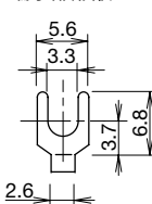
端子部形狀
