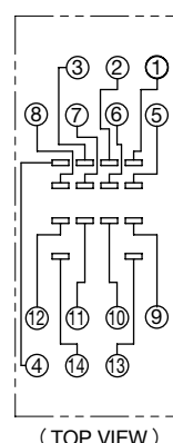
• 端子配置圖
