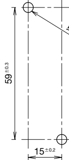
• 安裝孔加工圖
