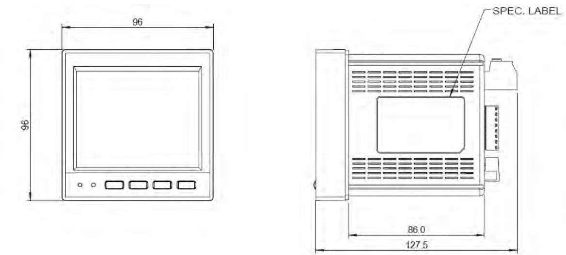
單位：毫米[英吋]
