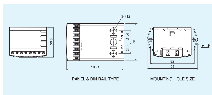
EOCR-3DM2 (過孔式)
