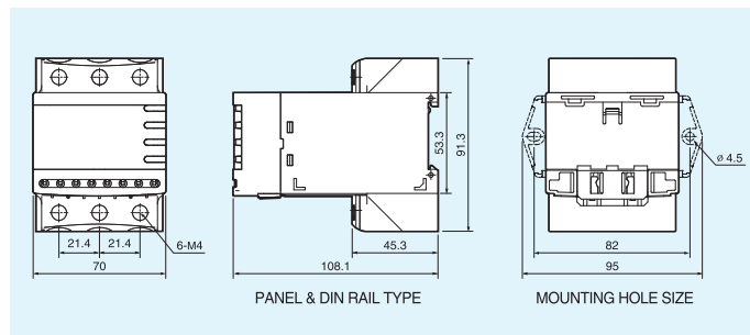
EOCR-3DM2 (端子式)
