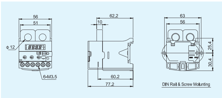
EOCR-SSD
