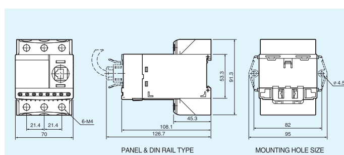
EOCR-FDM2 (端子式)
