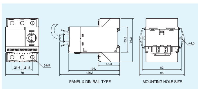
EOCR-iFDM (端子式)
