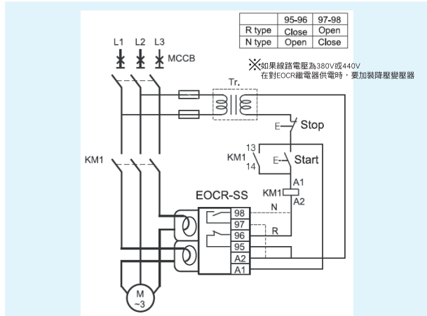
EOCR-SS
