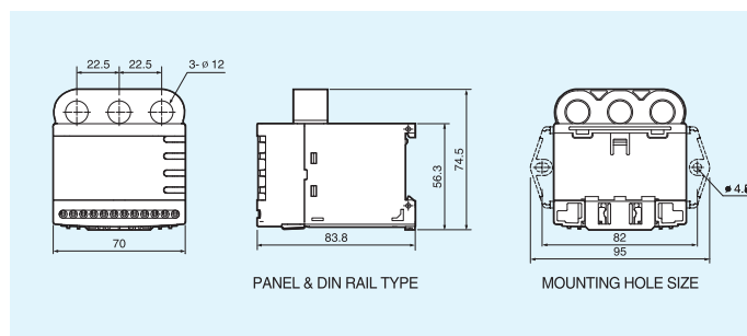
EOCR-i3DM (穿線式)
