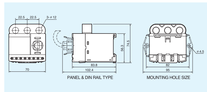
EOCR-FDM2 (穿線式)
