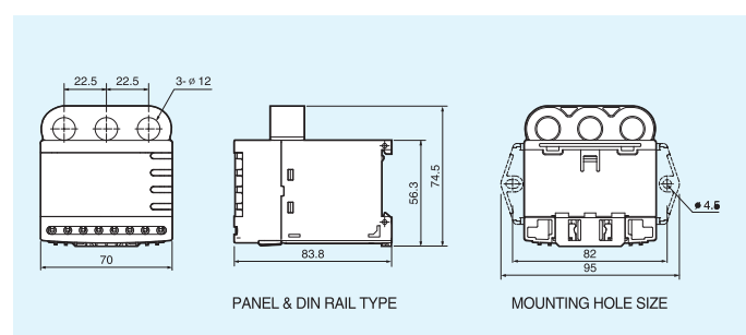
EOCR-3DM2 (穿線式)
