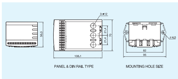
EOCR-i3DM (過孔式)
