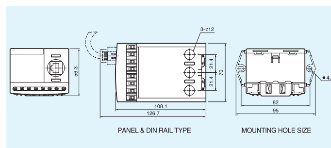
EOCR-FDM2 (過孔式)
