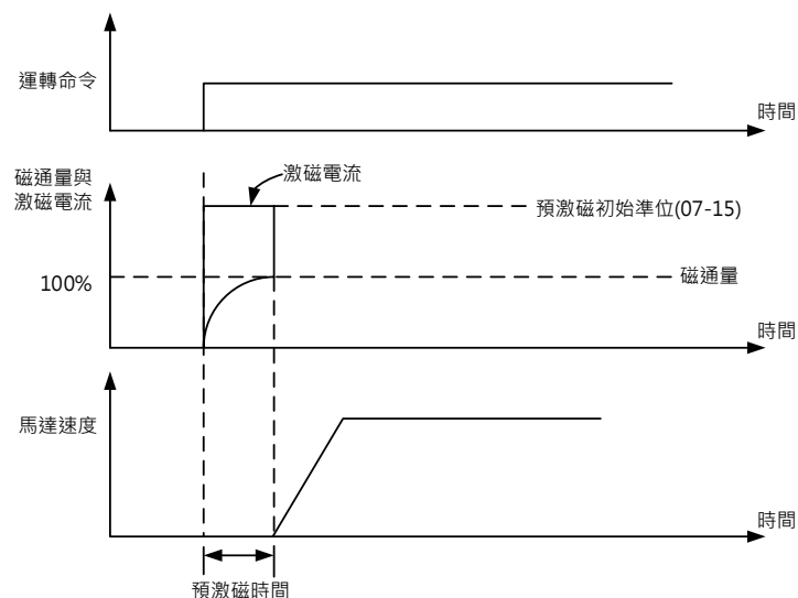
圖4.3.62 預激磁操作
