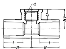
龍T接頭(塑膠牙)
