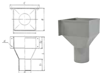
漏斗 Hopper 單位：mm
