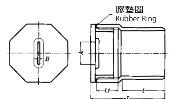
清除孔接頭 Cleanout Bushing 單位: mm
