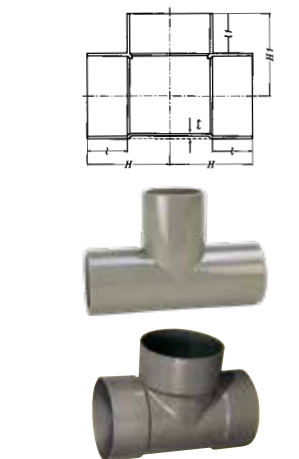
T 型同徑接頭 Tee
