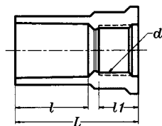
龍S接頭(塑膠牙)
