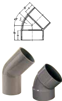
45° L 型接頭 45° Elbow
