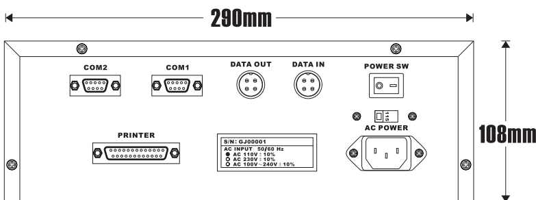
後視尺寸圖
