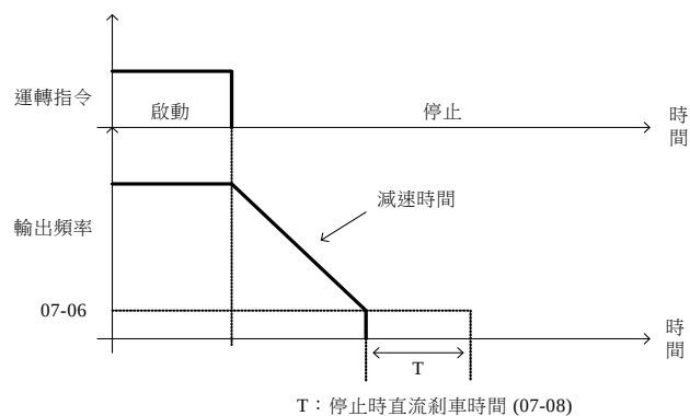
圖 4.3.58 減速停止
