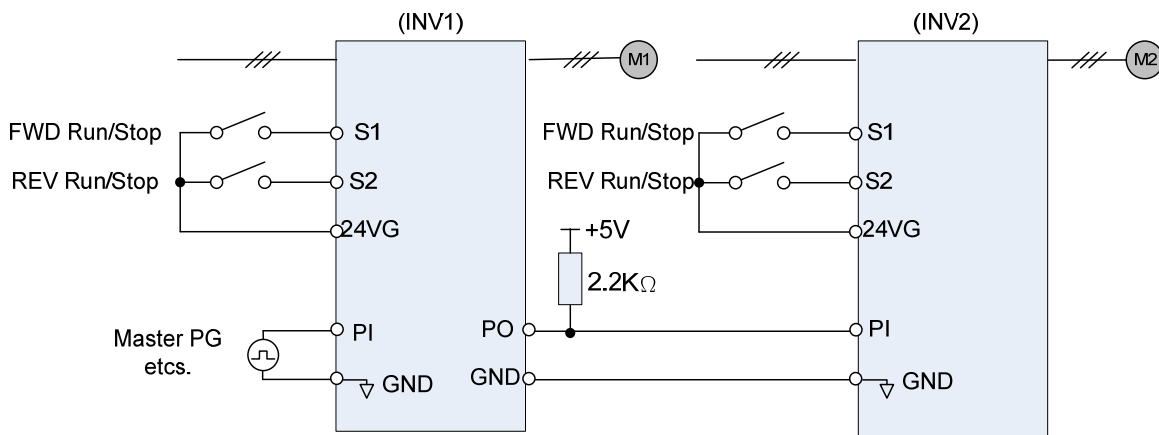
圖 4.3.32 2個轉換器連結操作
