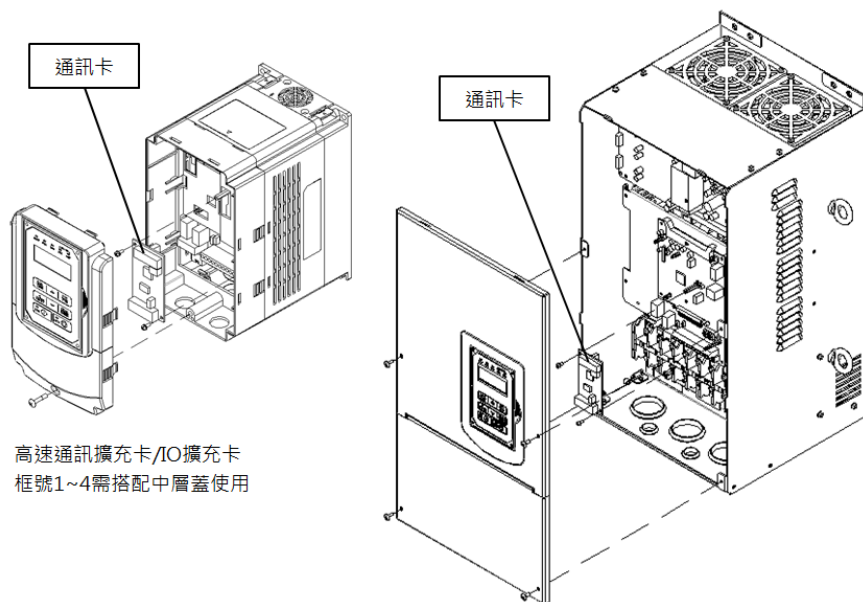
通訊卡安裝示意圖
