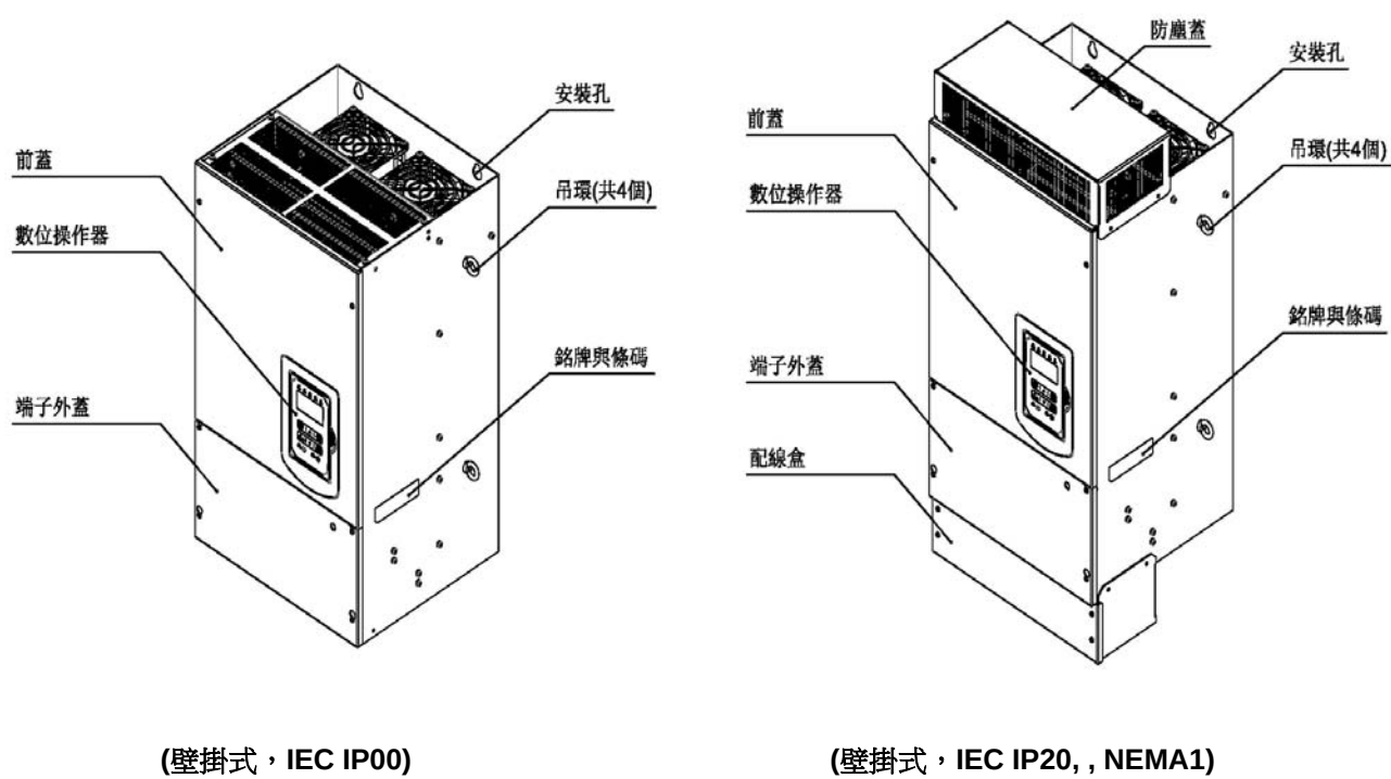
圖 3.2 A510s 外觀圖
