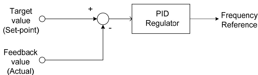
圖 4.3.28 PID控制
