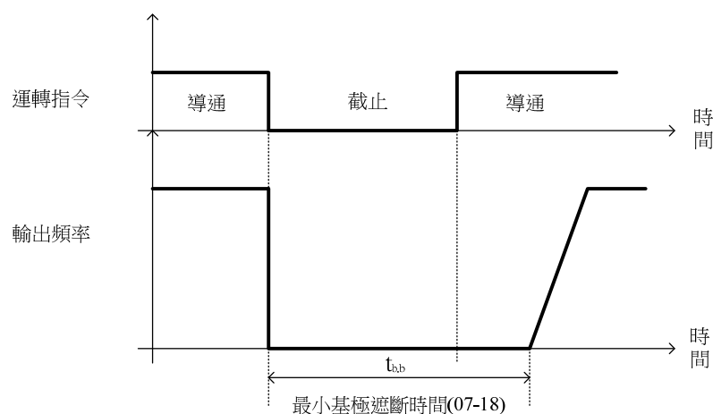
圖 4.3.59 自由運轉停止
