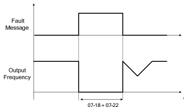
圖 4.3.55 自動復歸再啟動操作
