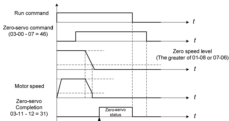
圖 4.3.97 零伺服操作
