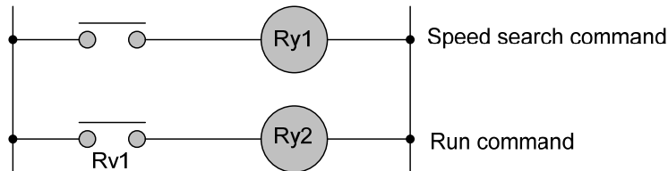
圖 4.3.64 速度搜尋及運轉命令
