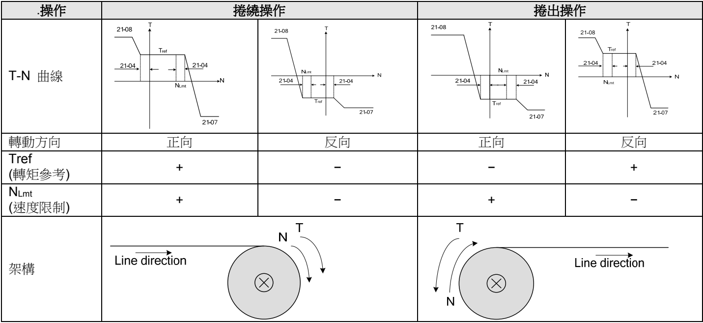
圖 4.3.130 捲繞和捲出操作
