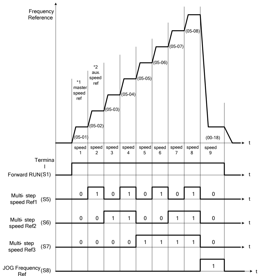
圖 4.3.18 9段速時序圖
