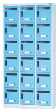
(117-5) DF-MB-18C ※訂貨生產 W900 × D350 × H1802(mm) $25800
