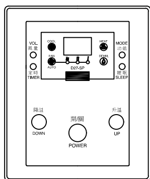
控制面板 120*100*16
