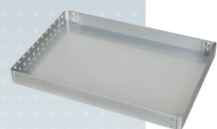
• KU-12 上層置物盒 (111-1) W710 × D490 × H65 (mm)
