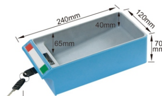
內部實際置放空間 W110 × D188 × H65~40 (mm)
