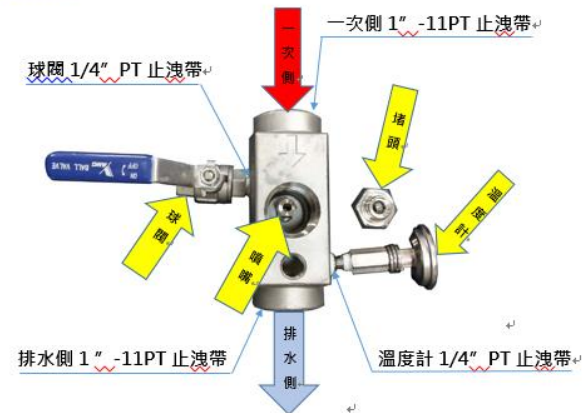
躍騰 DWS 9 祛水器 組裝說明
