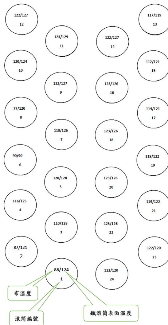
滾筒乾燥機溫度分佈圖
