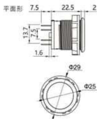
外型尺寸圖mm
