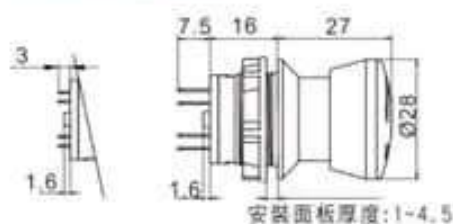
外型尺寸圖mm
