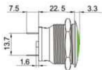
外型尺寸圖mm
