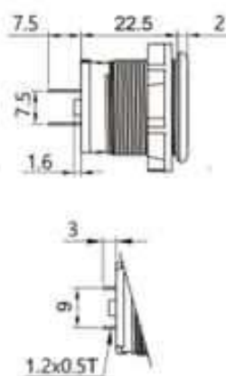
□最小安裝間距和安裝孔尺寸圖mm
