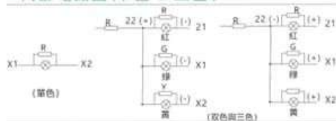
內部電路圖(單色 & 三色)
