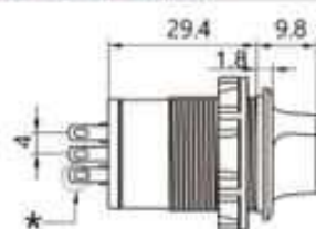
外型尺寸圖mm
