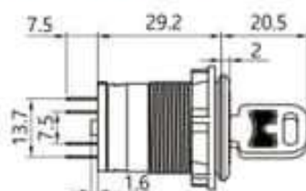
外型尺寸圖mm
