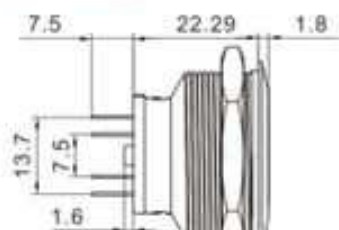
外型尺寸圖mm
