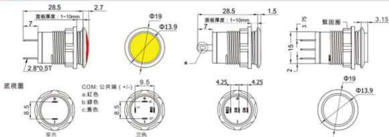
外型尺寸圖mm
