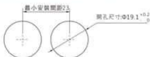
最小安裝間距和安裝孔尺寸圖mm
