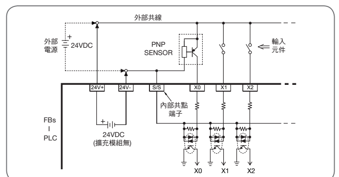
24VDC單端共點SOURCE輸入接線
