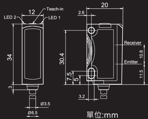
尺寸圖
