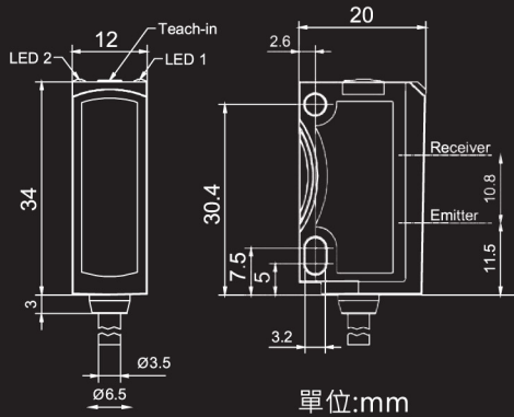
尺寸圖
