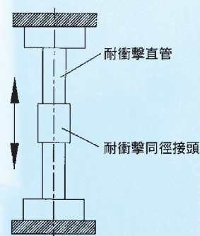
管體與接頭接合伸延試驗機
