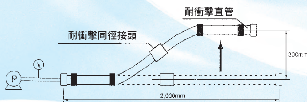
管體剪斷試驗機
