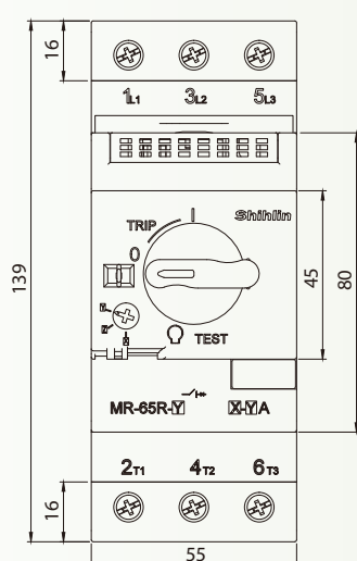
電動機保護斷路器 (旋鈕式) MR-65R
