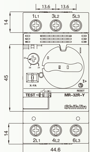
電動機保護斷路器 (旋鈕式) MR-32R
