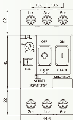
電動機保護斷路器 (按鈕式) MR-32S
