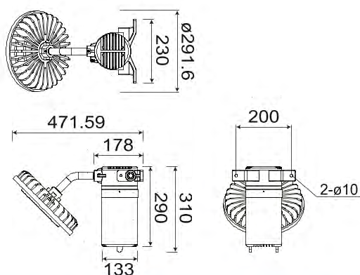
FP5壁掛型
