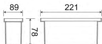
(預埋盒尺寸)
