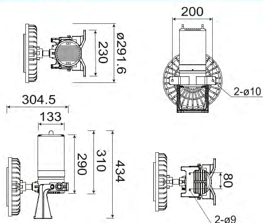
FP5投光型
