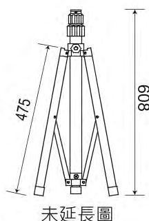
未延長圖
