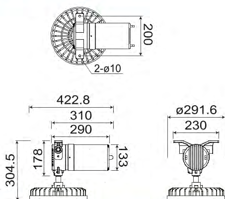
FP5壁掛型
