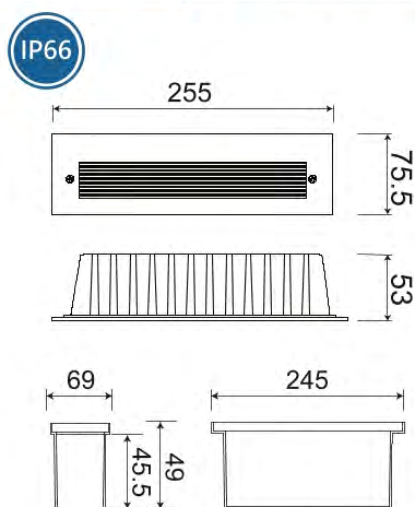
(預埋盒尺寸)
