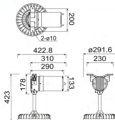
FP5投光型
