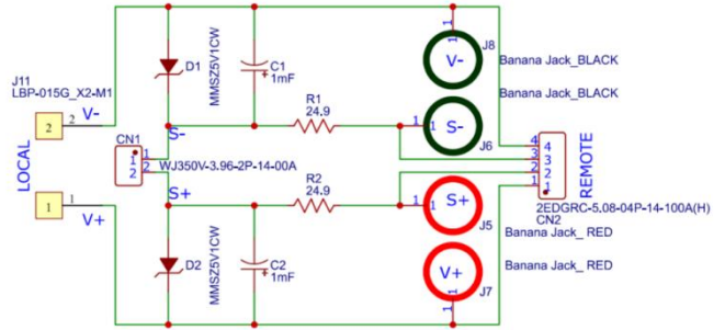
圖 14 遠端感應濾波器和 PWR-OPT05 原理圖
