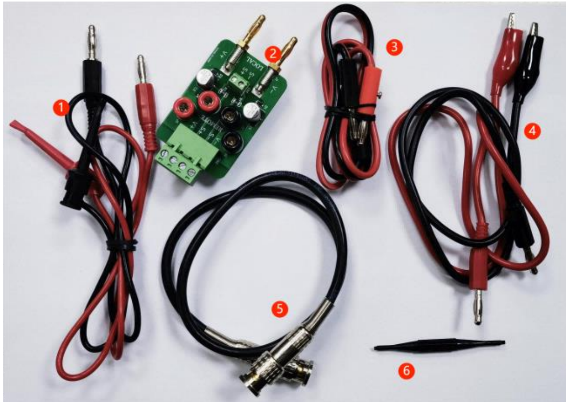
圖 2 PSRR 所需配件清單
