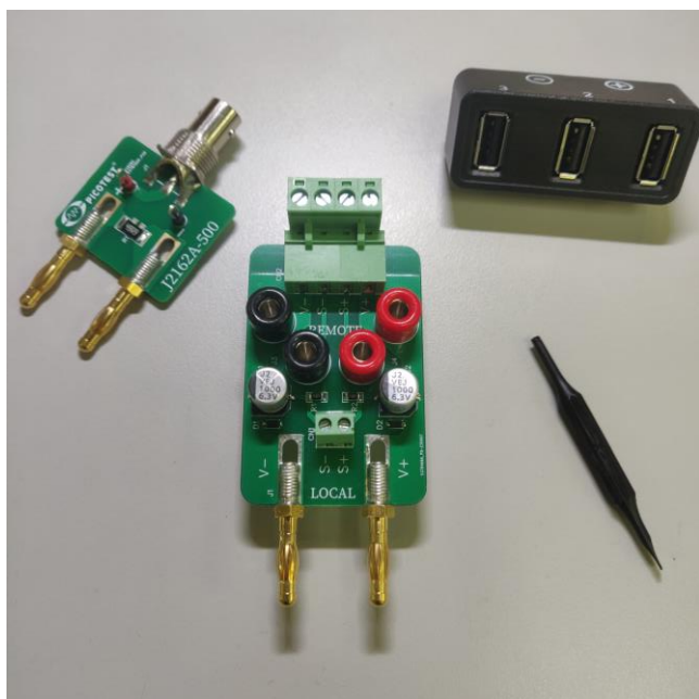
圖 2-1 J2122A 內含配件
