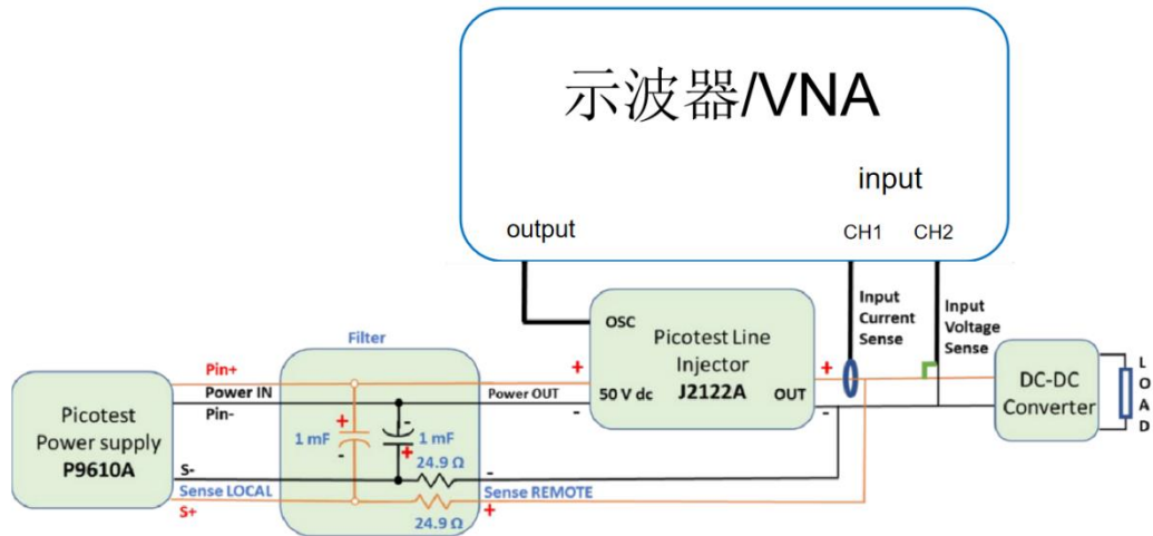
圖 12 利用遠端感應測量輸入阻抗的連接圖，以補償 J2122A 造成的壓降。由於 24.9 Ω 濾波電阻與內部電源分壓電阻串聯，因此會產生 75 mV 固定偏移。
