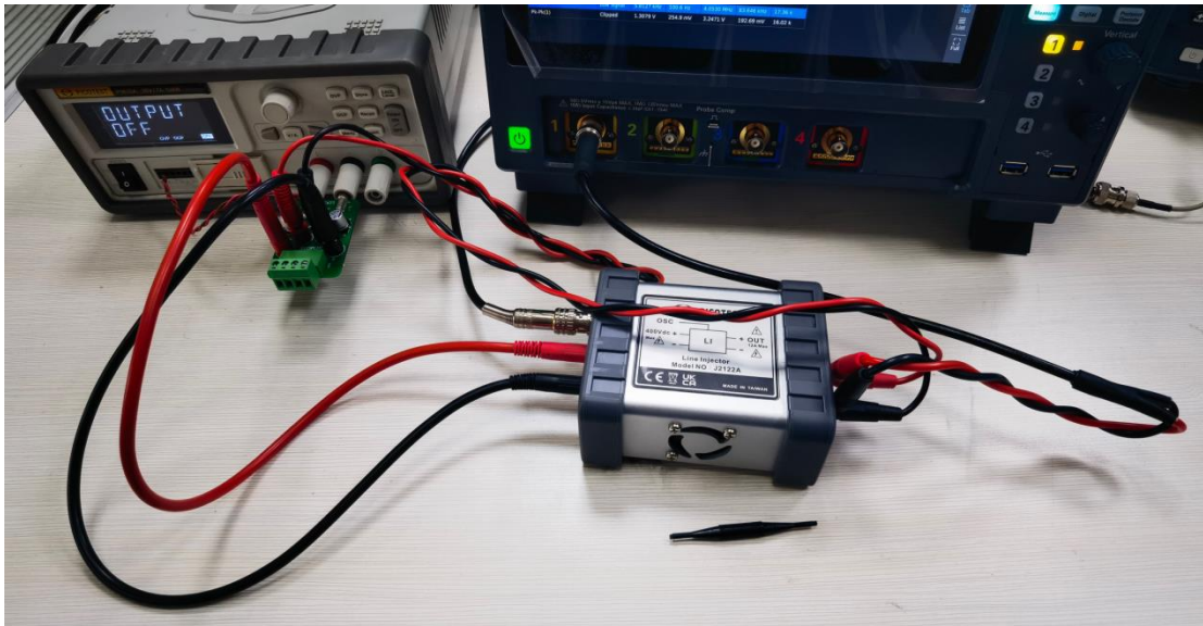
圖 15 使用 OPT05 連接示意圖
