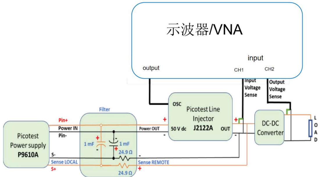
圖 13 利用遠端感應測量 PSRR 的連接圖，以補償 J2122A 引起的壓降。由於 24.9 Ω 濾波電阻與內部電源分壓器電阻串聯，因此會產生 75 mV 固定偏移。
