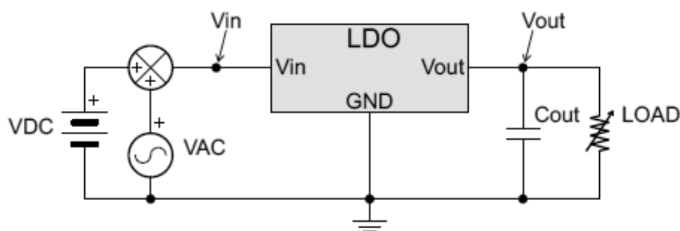
圖 1 低壓降穩壓器電源抑制比 (PSRR) 測量框圖
