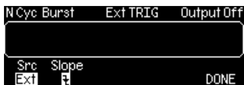
圖 4-17 Trig Setup 設定子目錄
