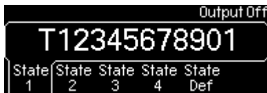
圖 5-5 “PowerOn” 子目錄
