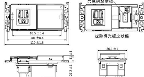
埋入式插座・三段調光腳燈組合 (附環境照度感測)
