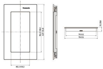
鋁合金 / 不繡鋼蓋板 (2連用)
