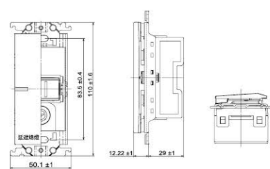
埋入式三段調光腳燈 (附環境照度感測)
