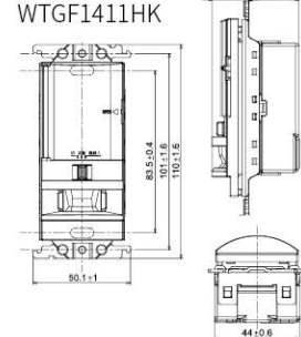
埋入式電子延遲熄燈開關B、埋入式洗手間開關
