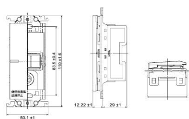
埋入式插座・三段調光腳燈組合 (附環境照度感測)
