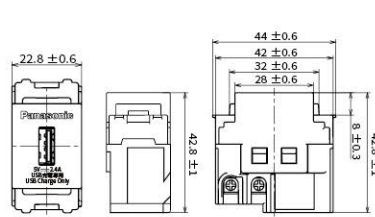
埋入式USB充電插座開關組合、埋入式USB智能快速充電插座開關組合、埋入式USB Power Delivery智能快速充電插座2孔・開關組合
