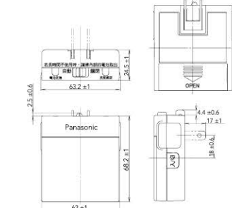
埋入式插座・三段調光腳燈組合 (附環境照度感測)
