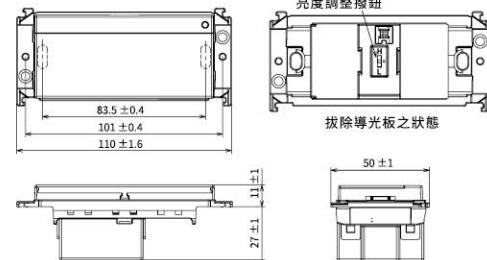
埋入式三段調光腳燈 (附環境照度感測)
