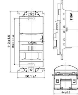
埋入式電子延遲熄燈開關B、埋入式洗手間開關
