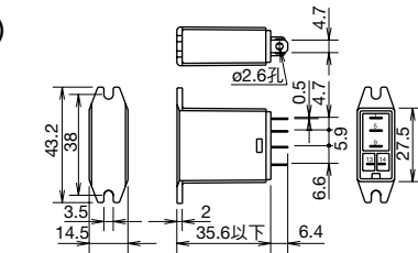
□SPDT 扁平端子型 (頂部凸緣安裝型)
