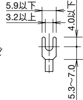
• 不能使用 R 形壓接端子
