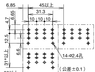
端子配置圖
