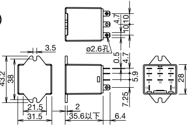
□3PDT 扁平端子型 (頂部凸緣安裝型)
