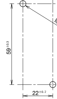
• 安裝孔加工圖
