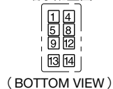
端子配置圖
