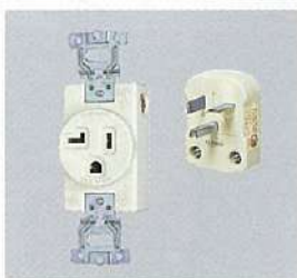
WFF3520 附接地極2P 20A 埋入式插座 20A 125V AC WFF5123 家用接地20A 彎角插座(125V) 20A 125V AC
