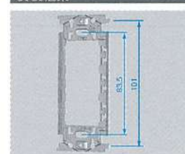
WNF3700 埋入安裝框架
