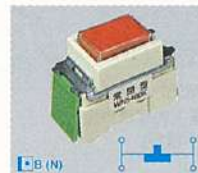
WN5460K-8 標名押釦B(B接點) 10A 300V AC ※可以表示負荷名
