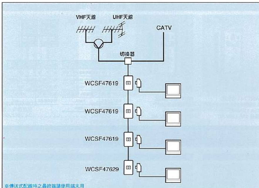
家用電視天線插座(U/V、CATV用)(5~1,000MHz)
