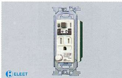
WN1741-832K EL保護附接地極插座 (附接地端子)(附門) 15A 110V AC 插座 15A 125V AC
