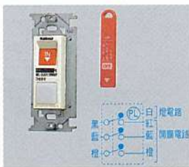
WNH5611-802 埋入式節能型鑰匙開關(客房用) (附位置顯示功能)(3路) 燈電路 10A 110V AC 開關電路 10A 250V AC(各電路)
