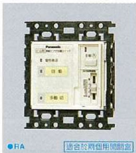
WN5600-832K 熱感自動開關(母器) (附信號輸出端子)3A 110V AC (檢測後連續動作時間，約10秒~30分鐘可調整型)
