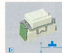
WN5401K-8 押釦B(單切) 10A 300V AC
