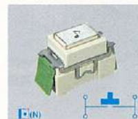
WN5461K-8 標名押釦B(單切) 10A 300V AC ※可以表示負荷名
