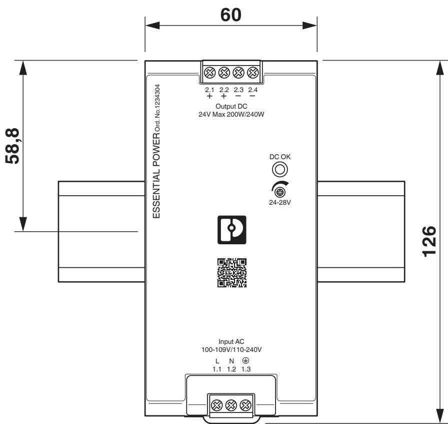
尺寸图
