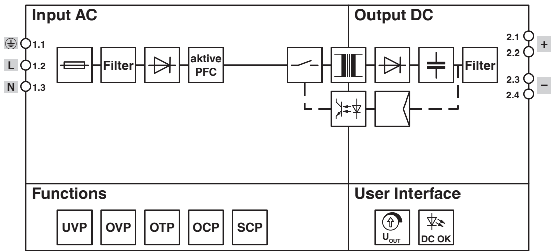
结构框图
