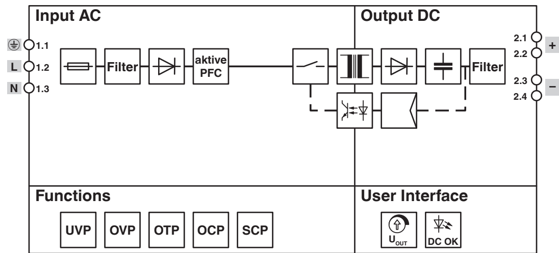
结构框图
