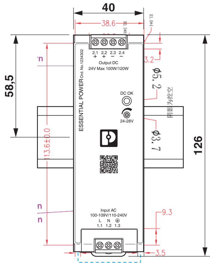
尺寸图
