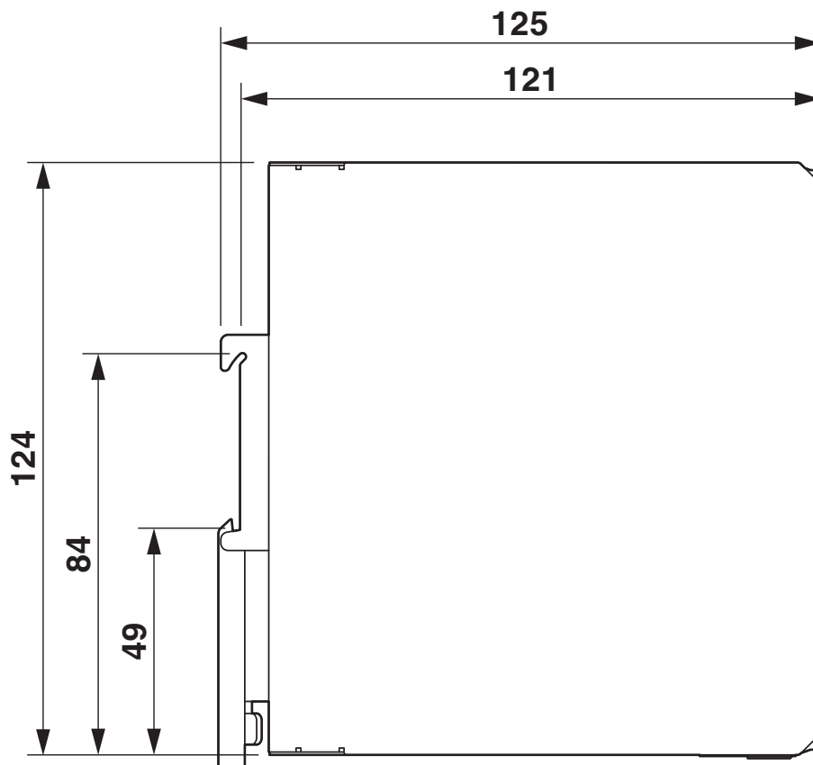
尺寸图
