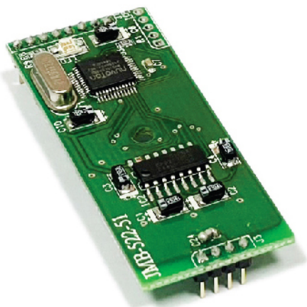
▲ JMB-522 (不含天線) 54(L)×22(W)×10(H)mm
