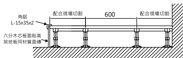
立面封板、牆面收邊示意圖
