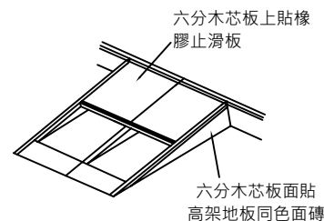
斜坡板示意圖
