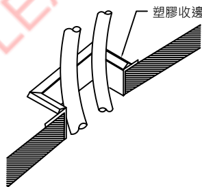
電纜線出口處開孔示意圖
