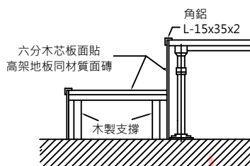
踏階及收邊示意圖
