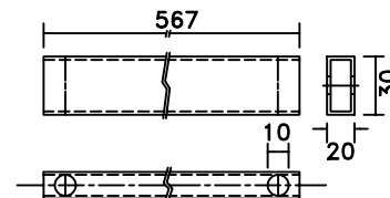
圖B 防震桁樑示意圖
