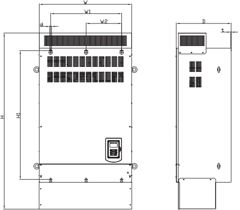
外型圖 G
